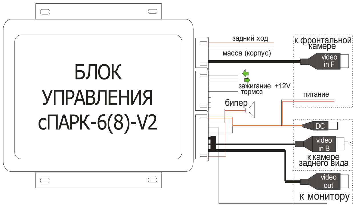
Схема подключений:
